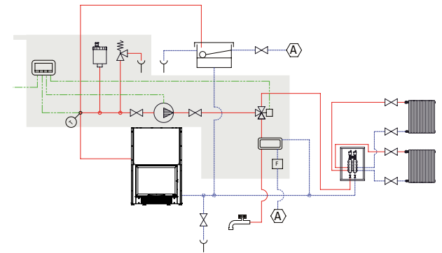
Kit camino ACS-VA + centralina. Accessorio Hydrotherm e Hydrosystem. ACS-VA Fireplace kit + control unit. Hydrotherm and Hydrosystem accessory. Kit cheminée ACS-VA + panneau de commande. Accessoire Hydrotherm et Hydrosystem. Bausatz Kamin ACS-VA + Steuergerät. Zubehör Hydrotherm und Hydrosystem. Kit chimenea ACS-VA + centralita. Accesorio Hydrotherm e Hydrosystem.
