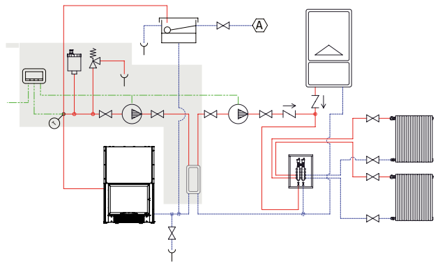
Kit camino-caldaia va + centralina. Accessorio Hydrotherm. VA Fireplace kit-boiler + control unit. Hydrotherm accessory. Kit cheminée-chaudière va + panneau de commande. Accessoire Hydrotherm. Bausatz Kamin-Kessel VA + Steuergerät. Zubehör Hydrotherm. Kit chimenea-caldera va + centralita. Accesorio Hydrotherm.
