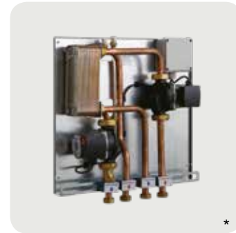
Kit camino-caldaia va + centralina. Accessorio Hydrotherm. VA Fireplace kit-boiler + control unit. Hydrotherm accessory. Kit cheminée-chaudière va + panneau de commande. Accessoire Hydrotherm. Bausatz Kamin-Kessel VA + Steuergerät. Zubehör Hydrotherm. Kit chimenea-caldera va + centralita. Accesorio Hydrotherm.
